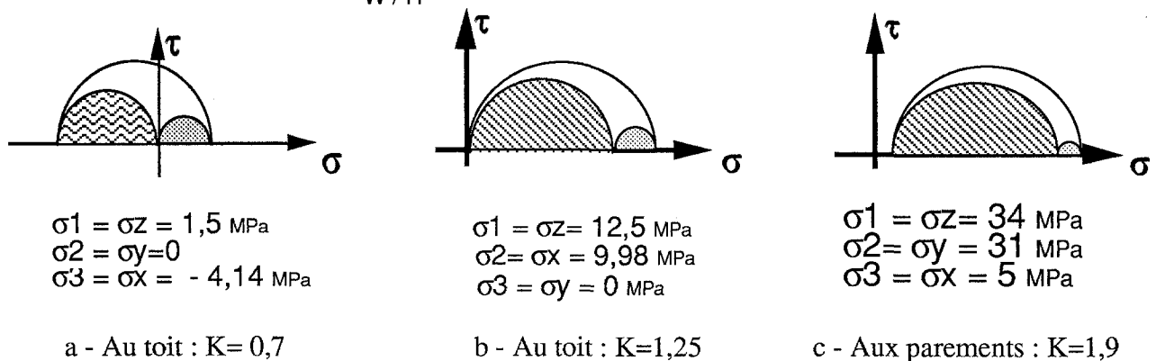
Fig 7 : Types de rupture d'une galerie rectangulaire (W/H=3) en fonction de rapport des contraintes verticale et horizontale ( \sigma_{y0} = 20 \text{ MPa} , compression positive)
