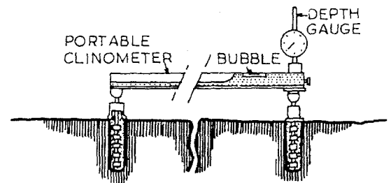
Figure 5 : Clinomètre portatif, [4]
