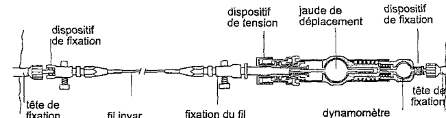
Figure 1: Le distomètre, un système mécanique très précis de mesure de convergence,
