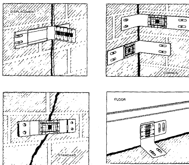
Figure 6 : Systèmes de mesure d'écartement de type "Vernier", [4]
