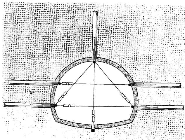
Figure 11 : Installation avec mesure de convergence entre les têtes d'extensomètres [4]
