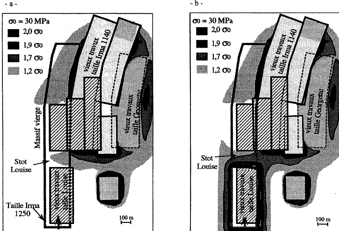
Figure 3 : a) Zones surcontraintes estimées par modélisation numérique avant l'exploitation de la taille Irma 1250 b) Zones surcontraintes normales estimées par modélisation numérique après 630 mètres de taille exploitée, le front d'exploitation est au niveau du stot de Louise.
