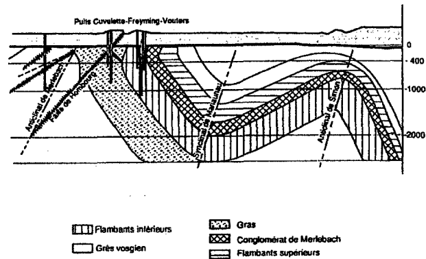
Figure 1 : Coupe géologique du bassin houiller lorrain
