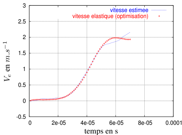
FIG. 6 – vitesses d'impact en force du temps
