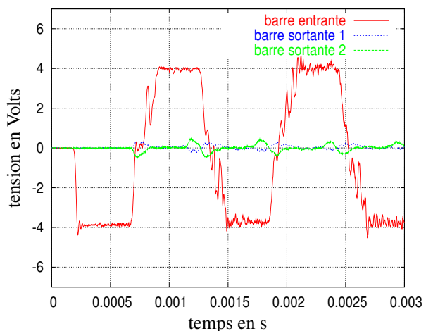
FIG. 2 – Signaux enregistrés
