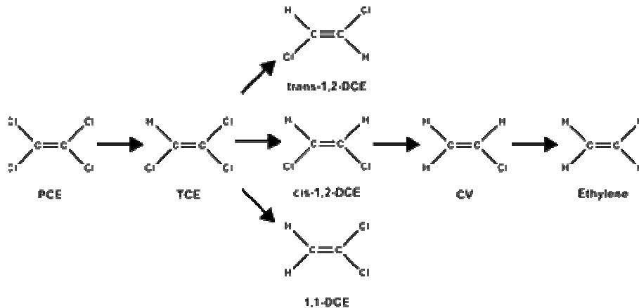
Figure 2 - Ensembles de réactions de dégradation du PCE dans les eaux souterraines par déchloration réductrice directe anaérobie [1]
