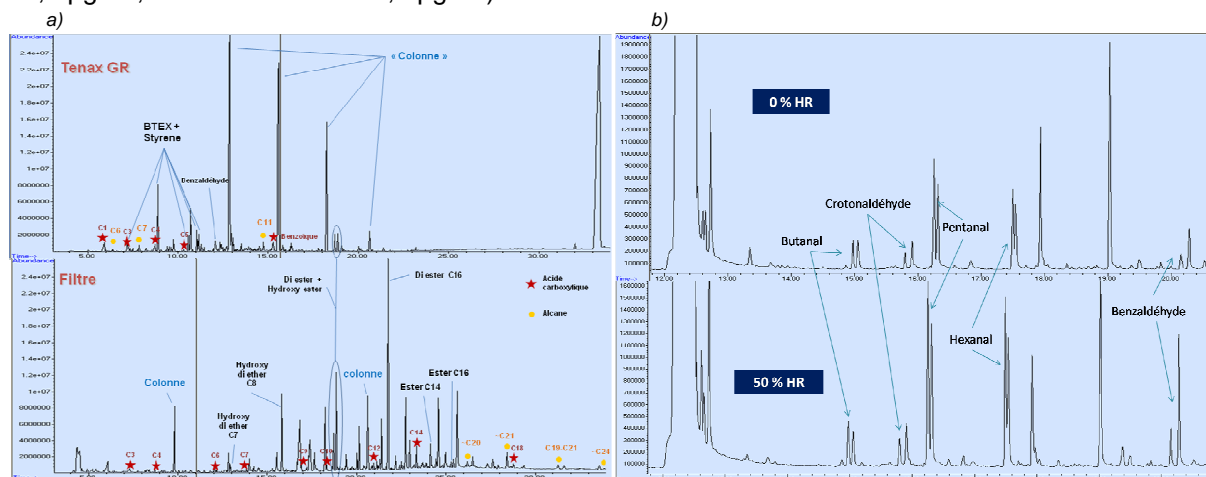
Figure 2 : Chromatogrammes obtenus a) lors du prélèvement en atmosphère réelle sur site INERIS, sans agent de dérivatisation (Tenax GR = phase gazeuse, Filtre = phase particulaire), b) lors de l'essai en atmosphère simulée d'aldéhydes gazeux à 0 et 50% d'humidité relative.
