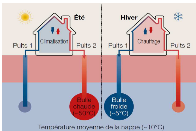
a) Schéma de principe d'un SETA
