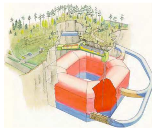
b) Cavité souterraine de Lyckebo en Suède (Hellström, 2012)
